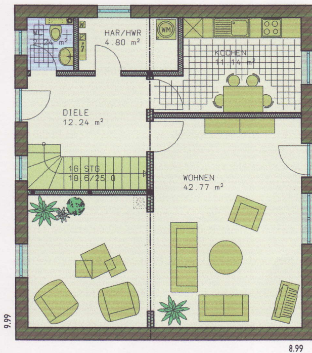
GRUNDRISS ERDGESCHOSS
