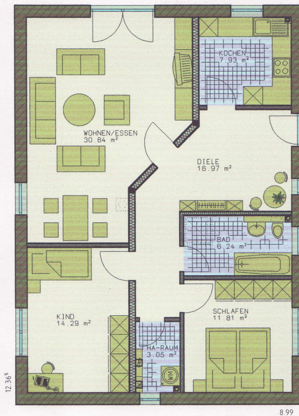
GRUNDRISS ERDGESCHOSS
