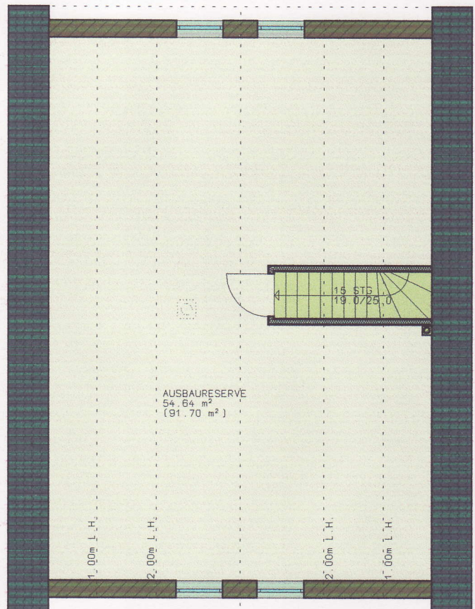
GRUNDRISS DACHGESCHOSS
